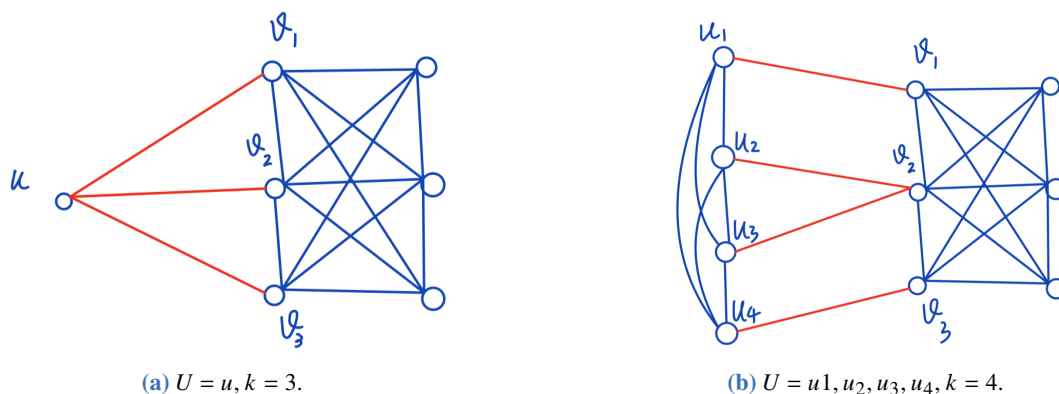
图 4.2: 顶点集 U 与 V - U 通过边割集 E' 相连.
